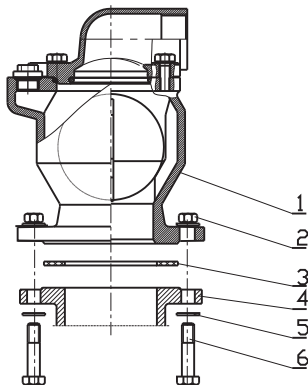
Схема монтажа
